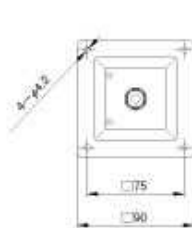
液晶モニター取付部寸法 (VESA75×75mmピッチ)
