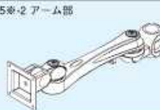
LA-50-2アーム部 寸法図
