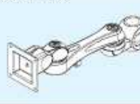
LA-50-6アーム部 寸法図
