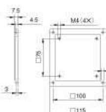
VESA100×100取付アダプタ(付属品) 寸法図
