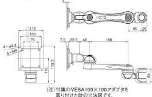
LA-50-6アーム部 寸法図
