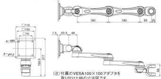
LA-50-6 アーム部
