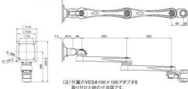
液晶モニター取付部寸法 (VESA75×75mmピッチ)
