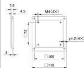
VESA100×100取付アダプタ(付属品) 寸法図
