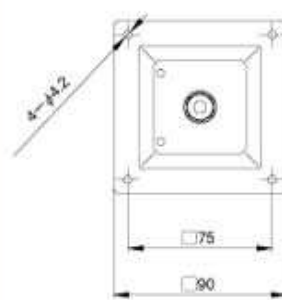
液晶モニタ取付部寸法 (VESA75×75mmピッチ)
