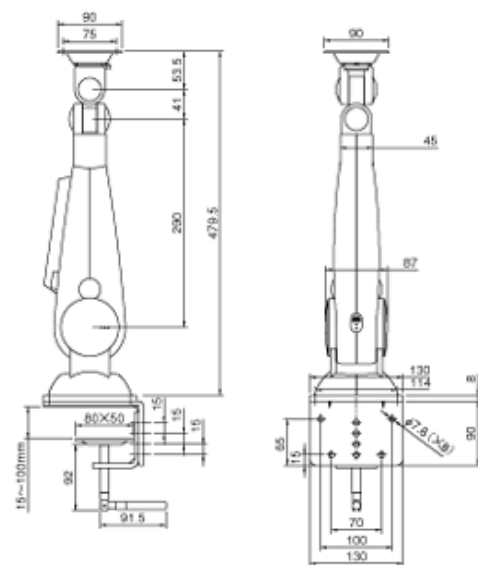
LA-31 寸法図
