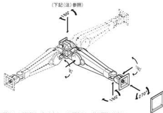
LA-35 可動範囲
