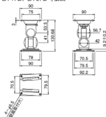
LA-17G、LA-37G 寸法図
