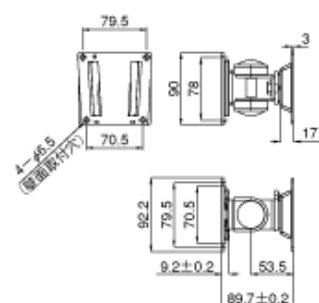
LA-16G 寸法図
