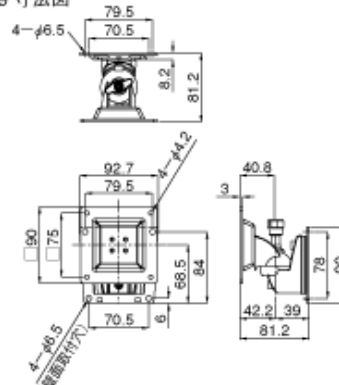
LA-19 寸法図
