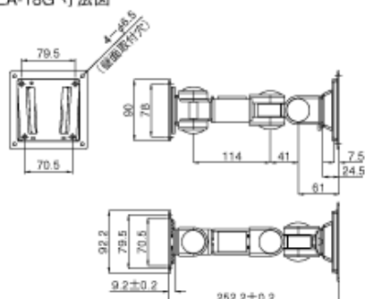
LA-18G 寸法図
