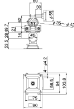
LA-16SN 寸法図
