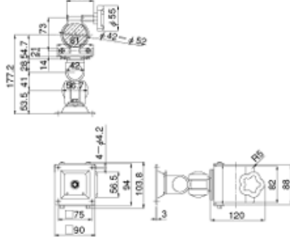
LA-37SN/37SW 寸法図
