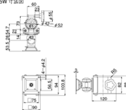
LA-16SW 寸法図
