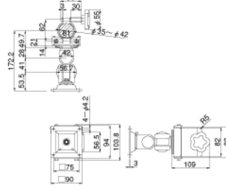
LA-17SN/17SW 寸法図
