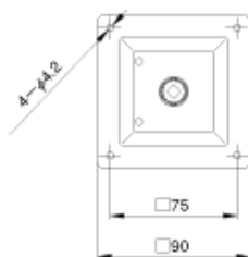
液晶モニタ取付部寸法 (VESA75×75mmピッチ)
