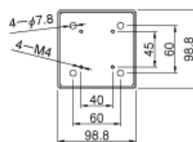
壁面取付部寸法図 (アーム底面の寸法図)
