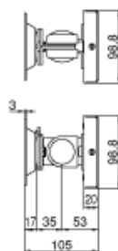
LA-16L 寸法図
