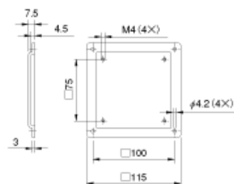
壁面取付部寸法図 (アーム底面の寸法図)
