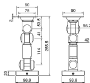
LA-18L 寸法図
