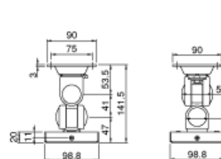
LA-17L/LA-37L 寸法図
