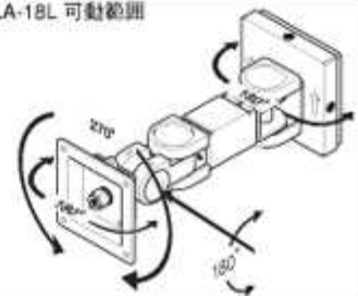
LA-18L 可動範囲
