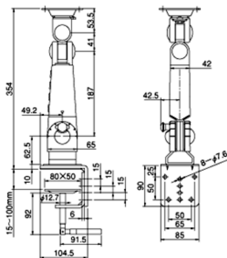
LA-11/LA-118K 寸法図
