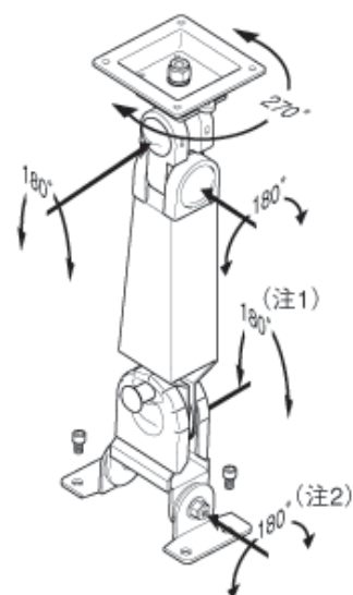
LA-12 可動範囲
